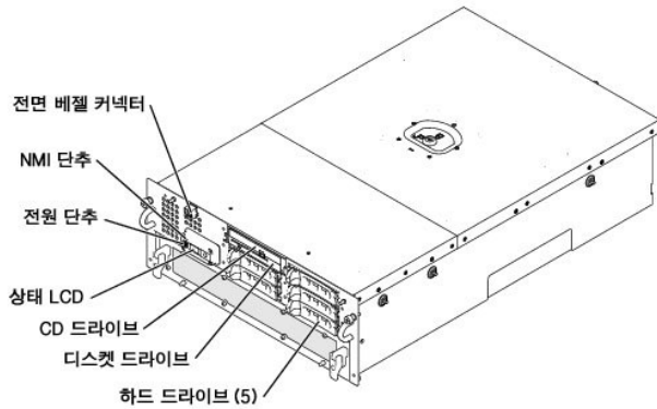
그림 1-2. 전면 패널 구조 및 표시등
