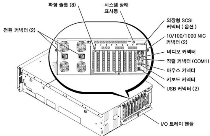
그림 1-4. 후면 패널 구조
