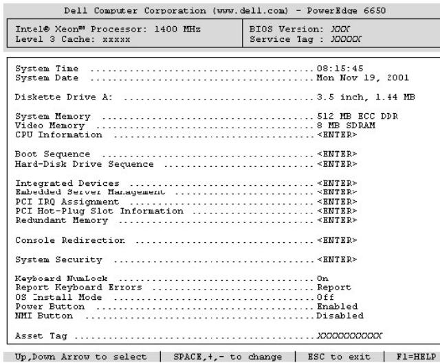
그림 3-1. 시스템 설치 프로그램 기본 화면
